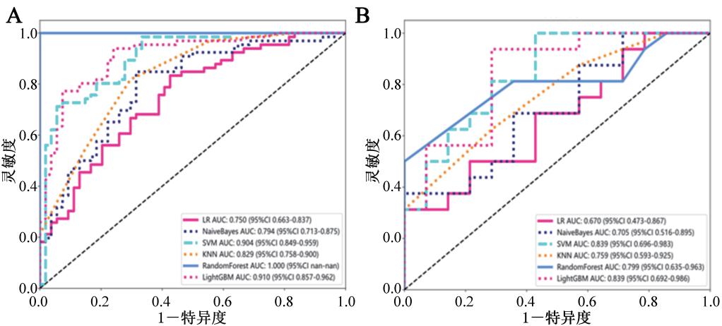
注：A 为训练集的 LR、NB、SVM、KNN、RF 和 LightGBM 的 ROC 曲线；B 为验证集的 LR、NB、SVM、KNN、RF 和 LightGBM 的 ROC 曲线。
