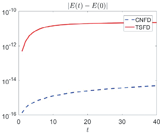
图 2 差分格式计算出的绝对能量差值
