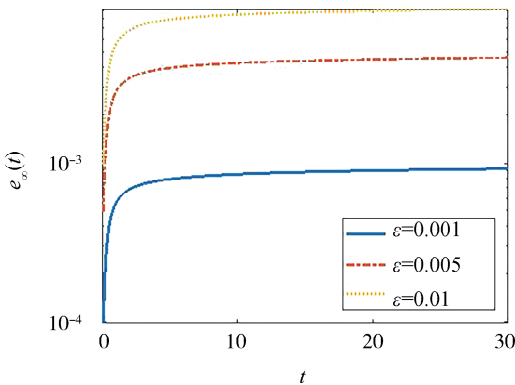
图 3 不同初值扰动下的误差演化
