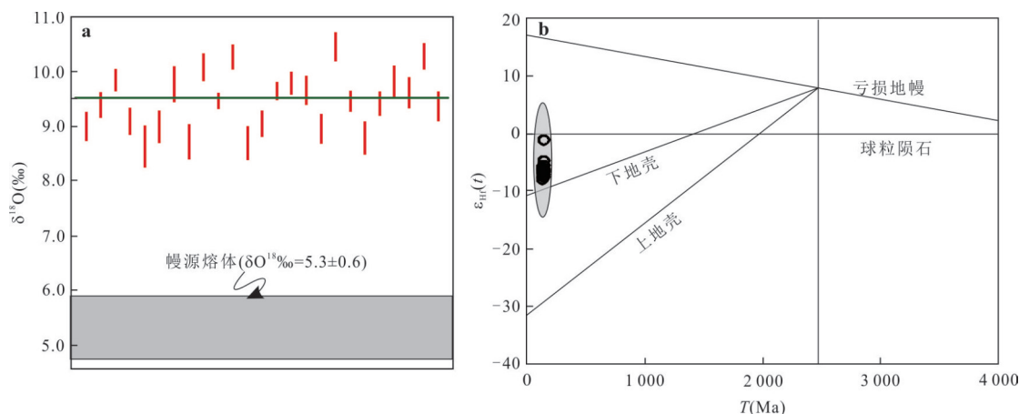
图 11 西山含榴英安岩 \delta^{18}\text{O}\text{‰} 加权平均图(a)和 \epsilon_{\text{Hf}}(t) - T(\text{Ma}) 图(b)
