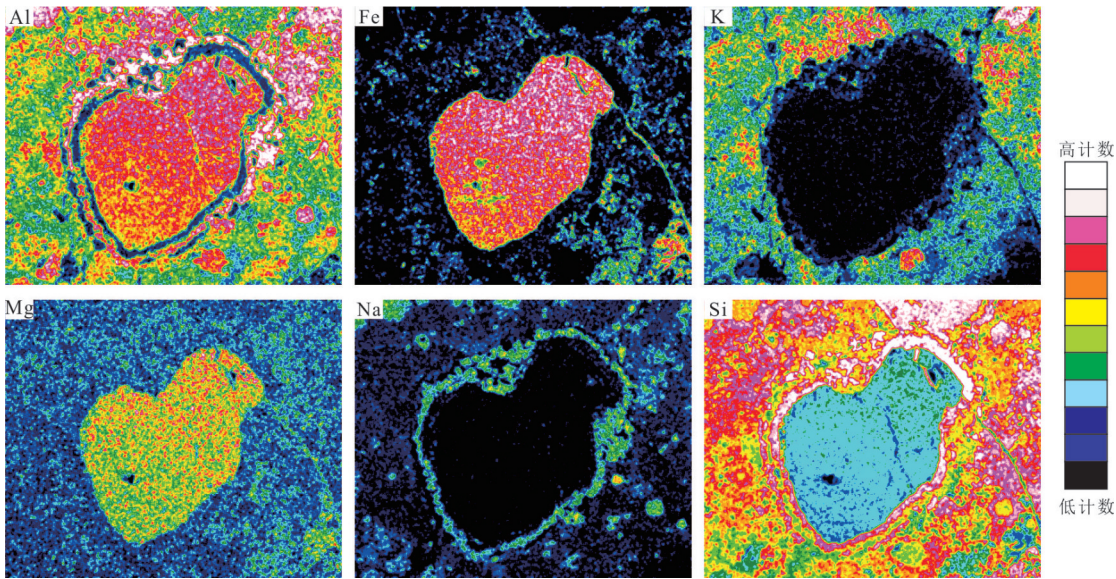
图8 类型Ⅲ石榴子石能谱面扫描元素分布图
