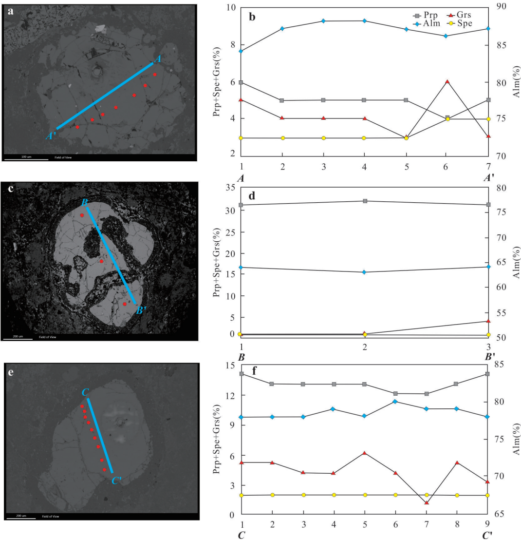
图3 西山含榴英安岩中3种类型石榴子石 EPMA 端元成分剖面图 Fig.3 EPMA composition profiles of typical magmatic garnets in the garnet-bearing dacite from Xishan complex a,b. 类型 I 石榴子石; c,d. 类型 II 石榴子石; e,f. 类型 III 石榴子石
