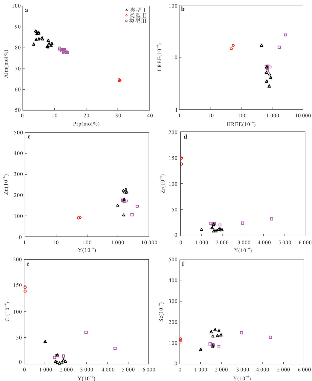
图5 西山含榴英安岩中3种类型石榴子石代表性稀土、微量元素二元图解
