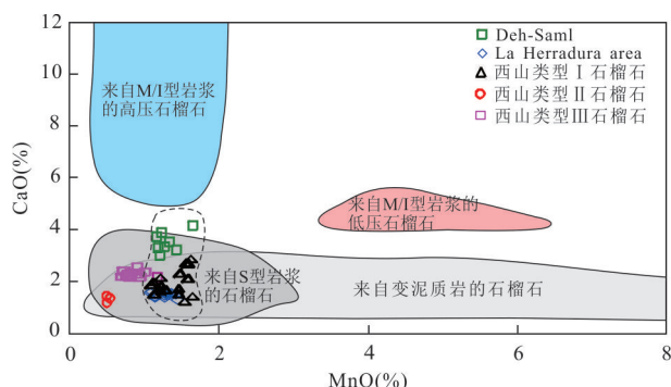
图12 石榴子石 MnO-CaO 二元图解
