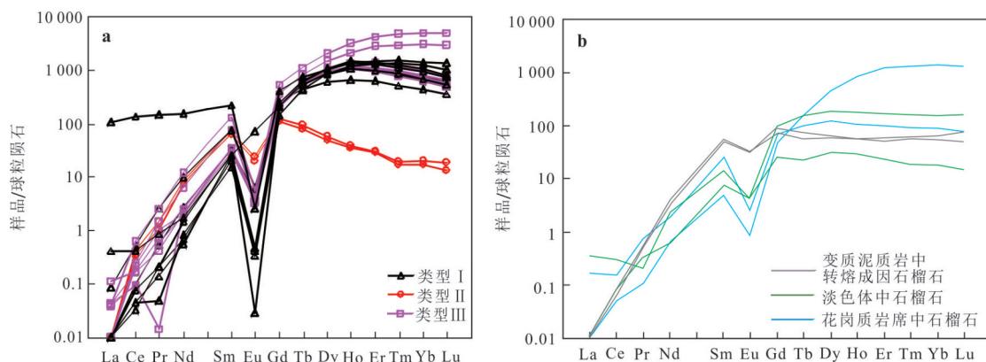
图4 西山含榴英安岩中3种类型石榴子石球粒陨石标准化稀土配分图(a)和斯威士兰姆洪多谷变质岩套中转熔成因石榴子石标准化稀土配分图(b)
