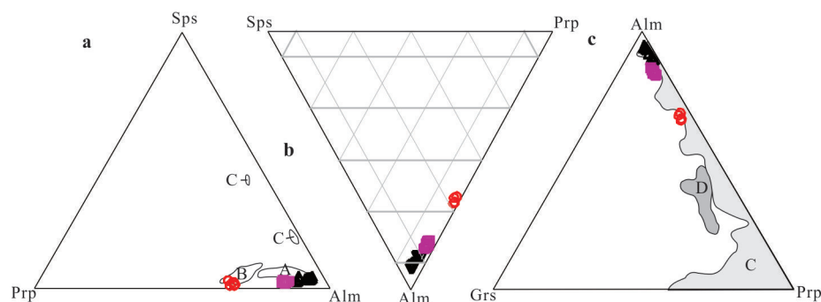
图10 石榴子石分类三角图
