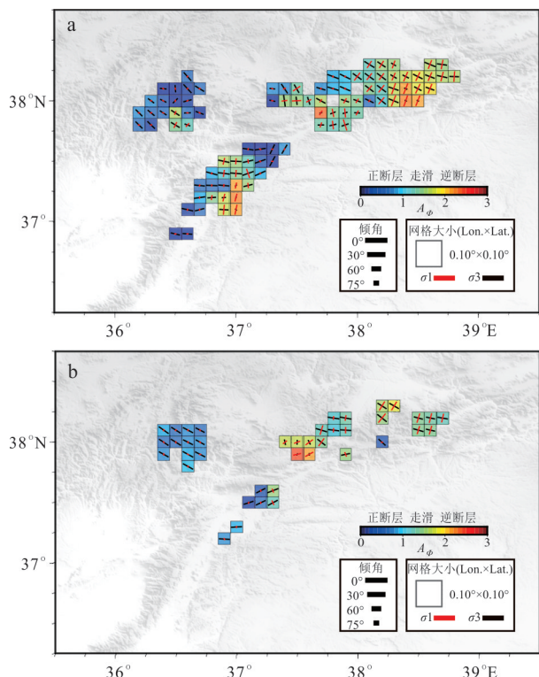
图4 基于POSE(a)与AFAD(b)震源机制解的应力场反演结果
