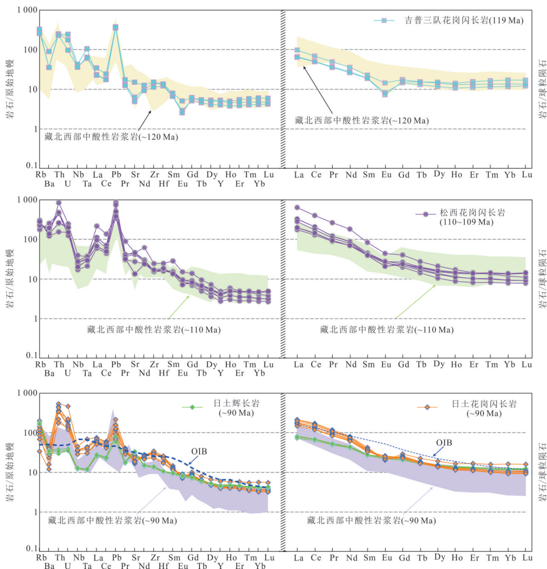
图5 藏北日土—松西地区岩浆岩原始地幔标准化多元素蛛网图与球粒陨石标准化稀土元素配分图
