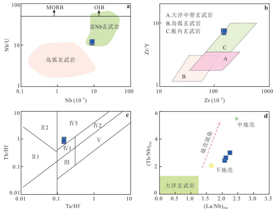
图 8 (a) Nb/U vs. Nb 图解; (b) Zr/Y vs. Zr 图解; (c) Th/Hf vs. Ta/Hf 图解; (d) (La/Nb)_{PM} vs. (Th/Nb)_{PM} 图解
