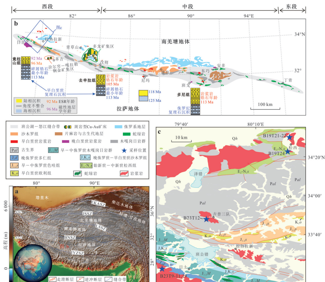
图1 (a)西藏及邻区构造格架简图(修改自 Fan et al. 2024a);(b)藏北西部地质简图(修改自 Hu et al. , 2022 and Zhang et al. , 2023)和(c)研究区松西、吉普三队和日土地区地质图
