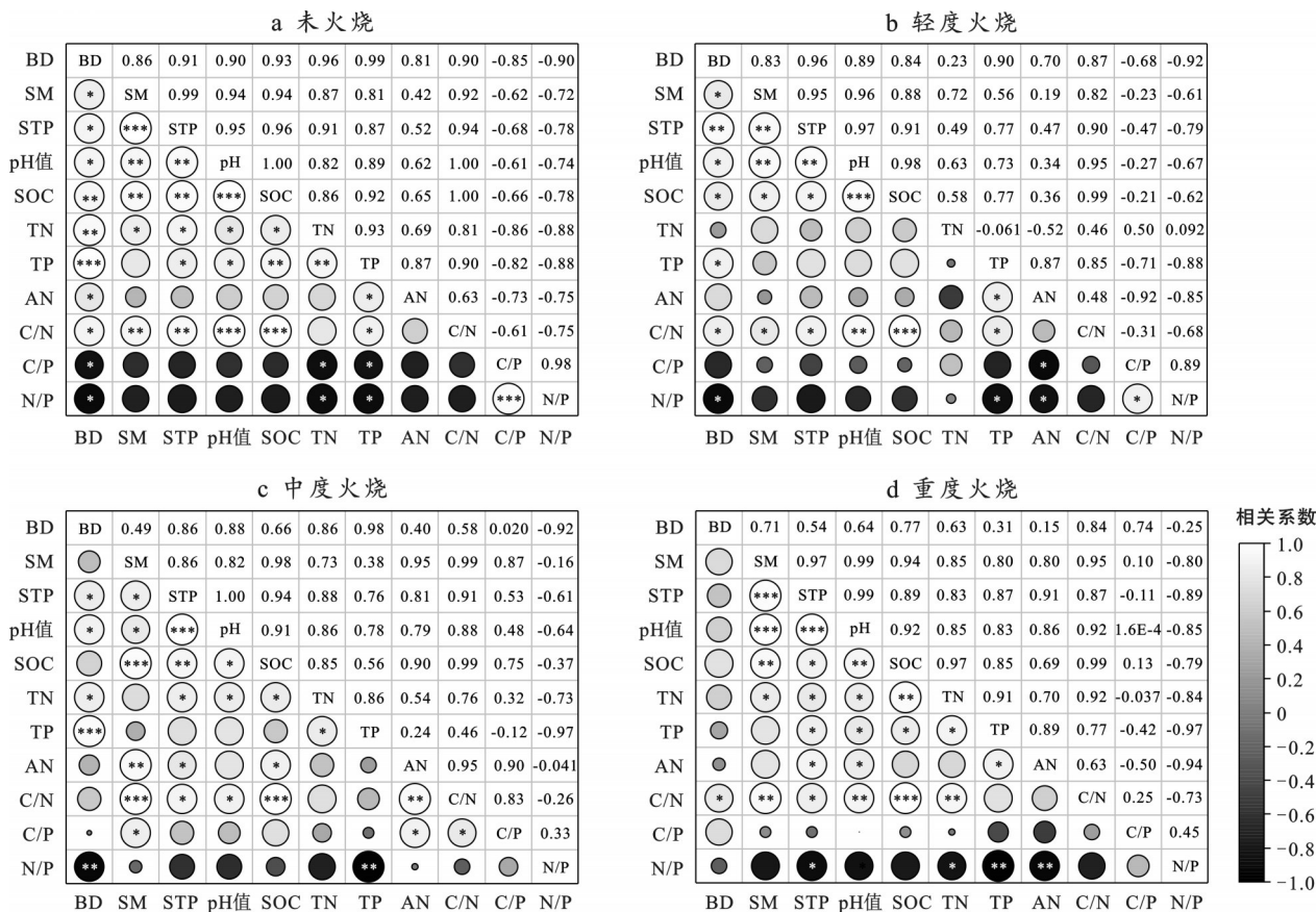
图4 不同火烧强度土壤理化性质与碳氮磷生态化学计量比之间的相关关系
