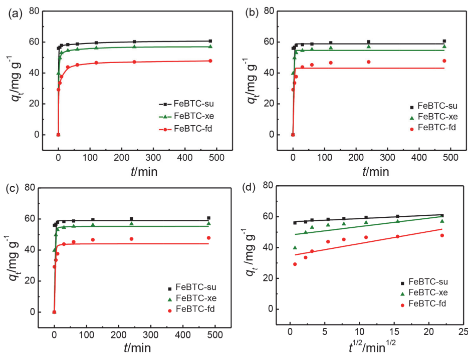
图9 FeBTC-su、FeBTC-fd和FeBTC-xe在303 K对 \text{Cr}_2\text{O}_7^{2-} 的(a) 吸附动力学曲线, (b) 准一级动力学模型, (c) 准二级动力学模型, (d) 颗粒内扩散模型
