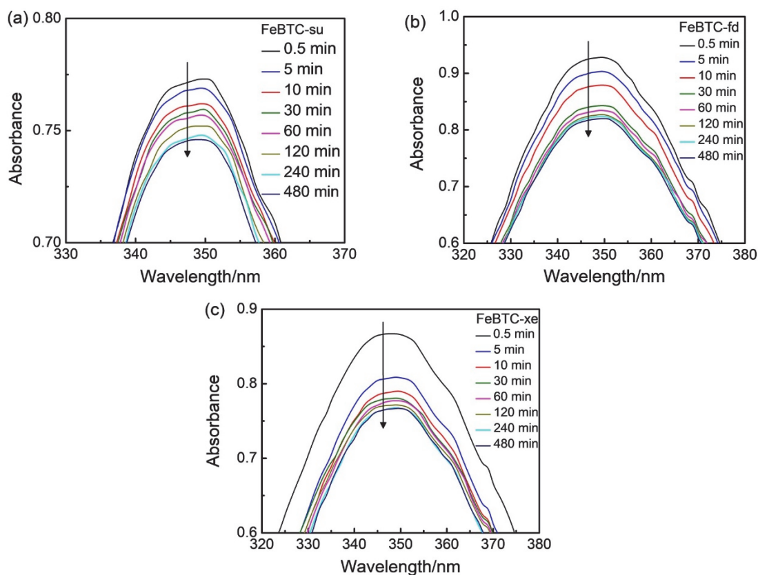
图8 (a) FeBTC-su气凝胶, (b) FeBTC-fd气凝胶和 (c) FeBTC-xe干凝胶对 \text{Cr}_2\text{O}_7^{2-} 吸附的紫外吸收光谱随吸附时间变化图
