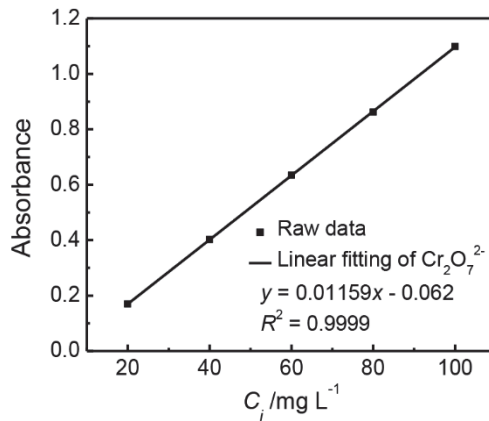
图5 \text{Cr}_2\text{O}_7^{2-} 的标准曲线
