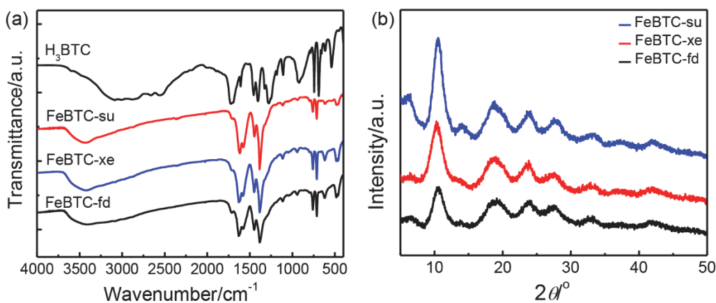
图6 (a) FeBTC-su气凝胶、FeBTC-fd气凝胶、FeBTC-xe干凝胶和 \text{H}_3\text{BTC} 的红外吸收光谱图; (b) FeBTC-su气凝胶、FeBTC-fd气凝胶和FeBTC-xe干凝胶的X射线粉末衍射图
