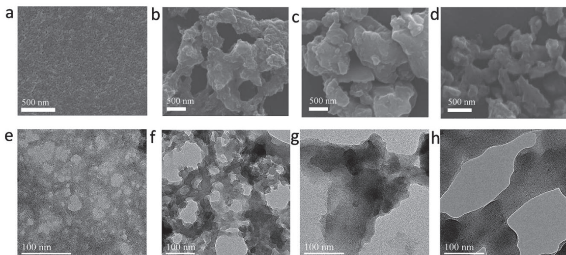
图3 (a) FeBTC湿凝胶、(b) FeBTC-su气凝胶、(c) FeBTC-fd气凝胶和(d) FeBTC-xe干凝胶的SEM形貌图，(e) FeBTC湿凝胶、(f) FeBTC-su气凝胶、(g) FeBTC-fd气凝胶和(h) FeBTC-xe干凝胶的TEM形貌图
