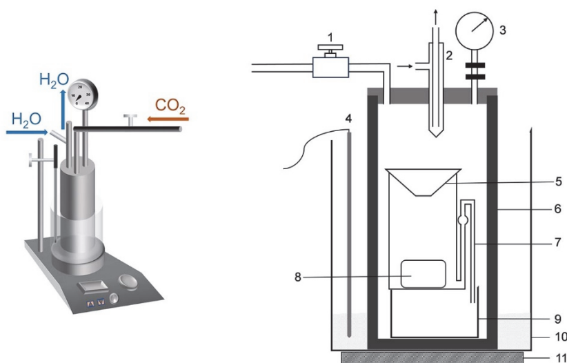
图2 亚临界干燥装置示意图
