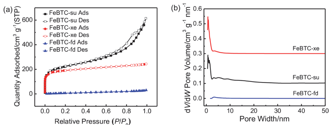
图7 (a) 77 K下FeBTC-su气凝胶、FeBTC-fd气凝胶和FeBTC-xe干凝胶的 N_2 吸附-脱附等温线; (b) 通过非局域密度泛函理论计算的孔径分布
