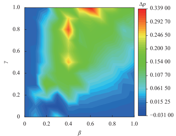
a. \Delta p - (\beta, \gamma) 的二维相图
