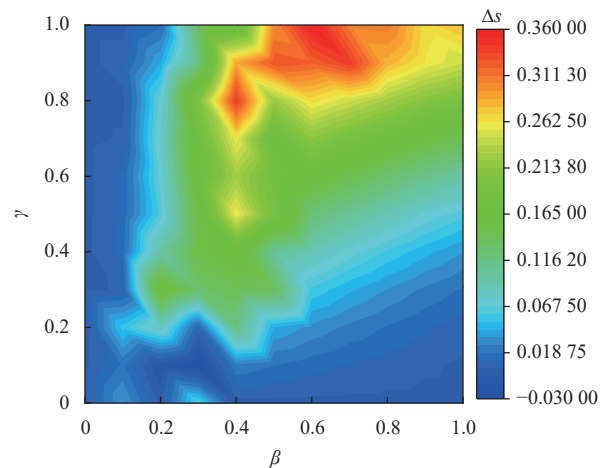
b. \Delta s - (\beta, \gamma) 的二维相图
