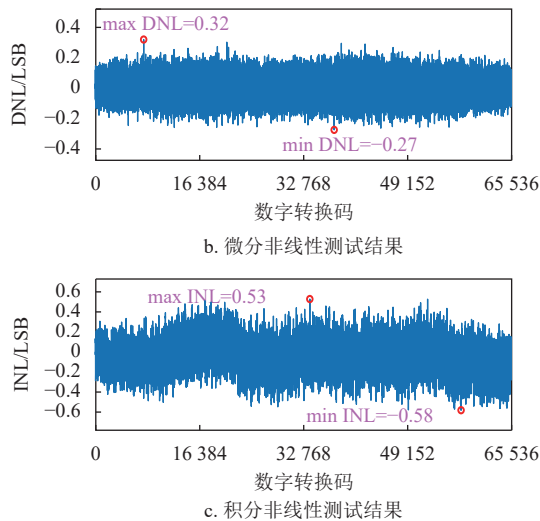
图 12 ADC 动态性能及直流线性度
