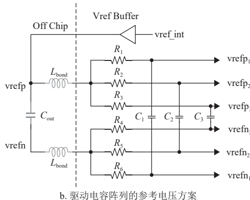
图 5 电容阵列结构及其参考电压驱动方案
