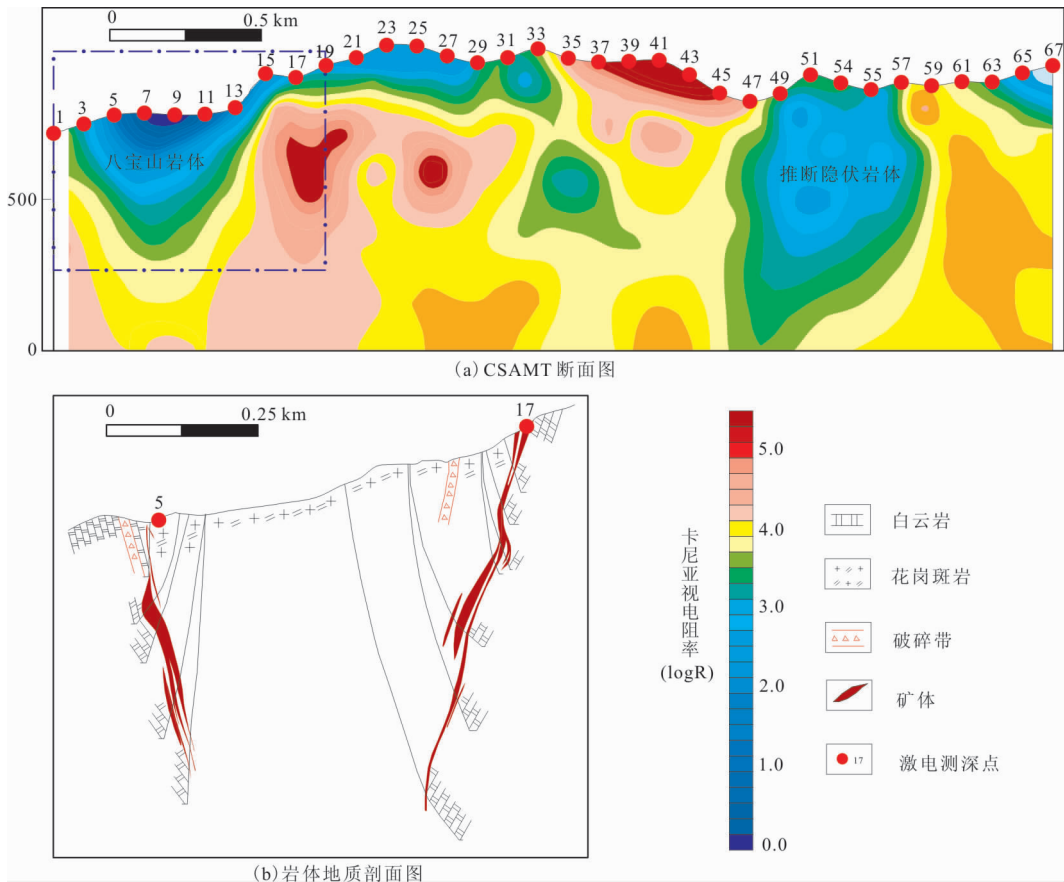
图7 CSAMT 断面图及岩体地质剖面图
