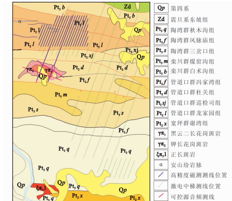
图4 八宝山矿区及其外围综合地球物理勘查工程布置图
