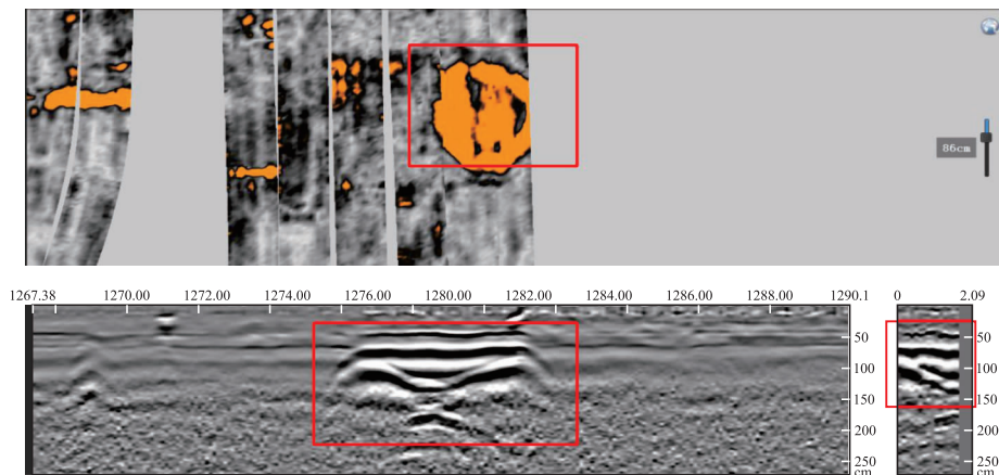
图 12 三维地质雷达空洞图谱
