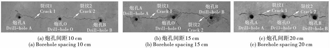
图3 三孔爆破实验结果图
