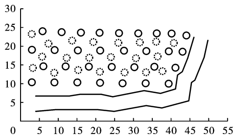
图6 炮孔布置图(单位:m)
