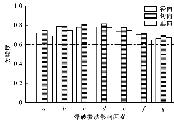
图 3 关联度结果
