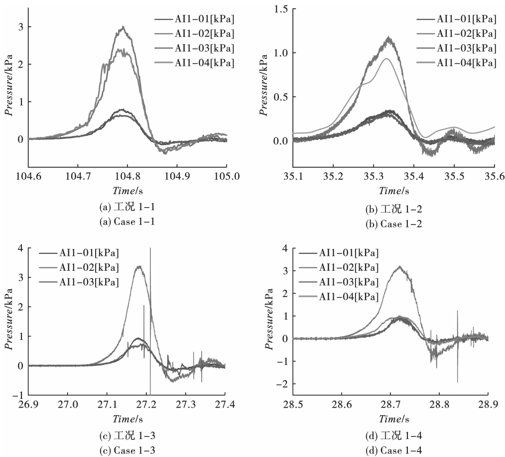
图 8 1 m 3 甲烷爆炸荷载时程曲线
