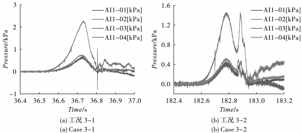
图 10 27 m 3 甲烷爆炸荷载时程曲线
