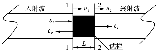
图 3 SHPB 实验原理简图
