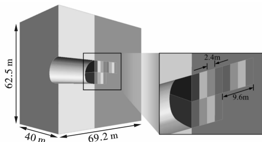
图8 台阶法隧道爆破开挖数值模型
