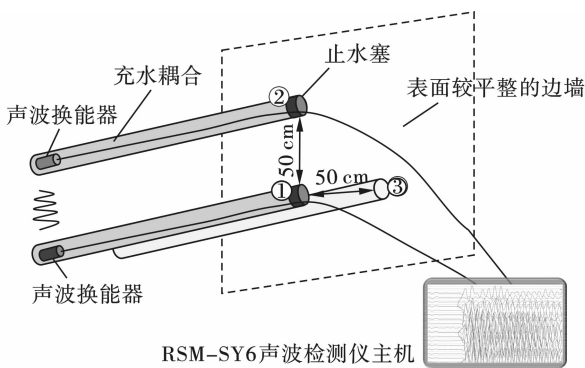
图3 声波测试方案图
