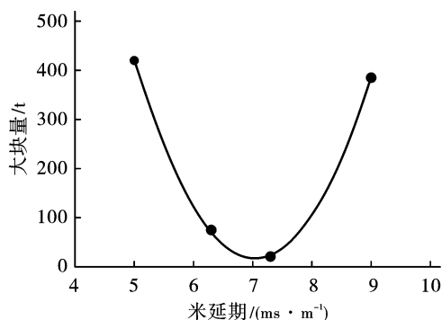
图8 每米延期时间与岩石破碎效果关系
