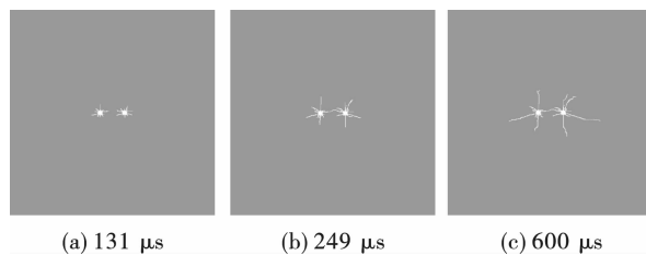
图 11 t = 131 \mu\text{s}, 249 \mu\text{s}, 600 \mu\text{s} 切缝角度
