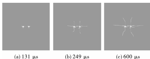
图 12 t = 131 \mu\text{s}, 249 \mu\text{s}, 600 \mu\text{s} 增设空孔双孔
