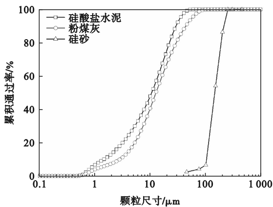
图 2 ECC 基体材料粒径分布
