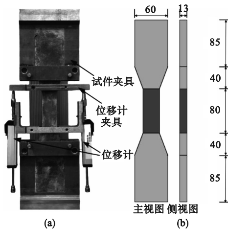
图 4 直接拉伸试验装置及试件尺寸(单位:mm)
