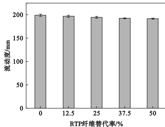
图 5 不同 RTP 纤维替代率的 ECC 流动度
