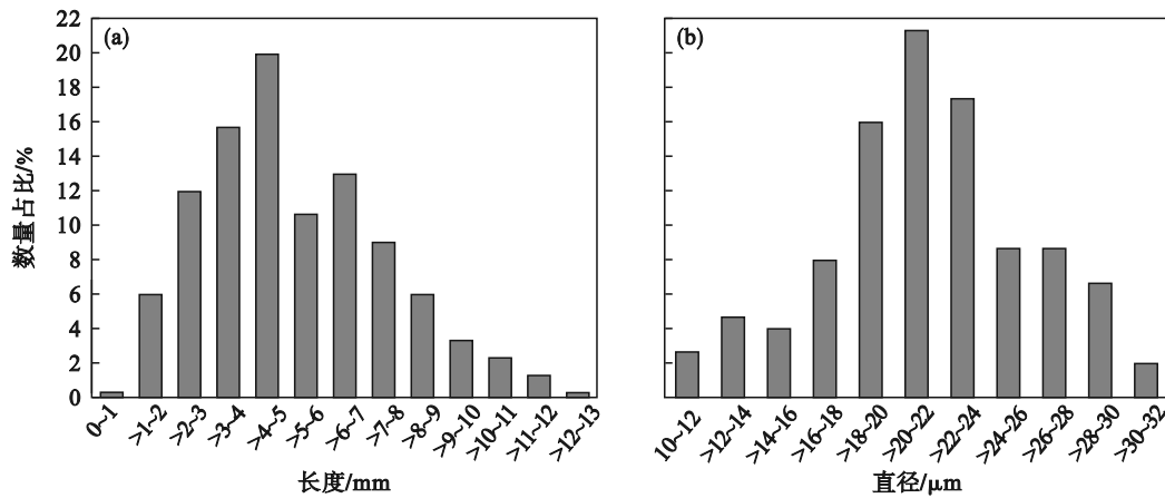
图 3 RTP 纤维长度与直径分布图
