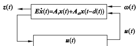
图 1 闭环控制系统结构图
