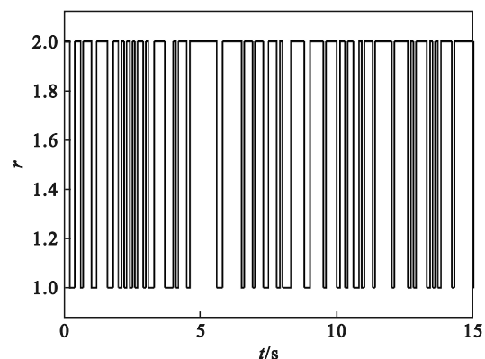
图 3 系统模态 r(t) 的轨迹
