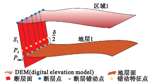
图 5 断层错动隐式点计算原理
