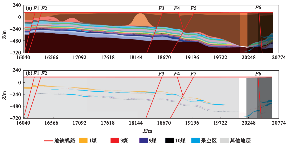
图11 地铁线路剖面
