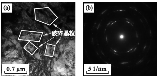
图 12 镍基单晶高温合金多晶化形貌和结构衍射
