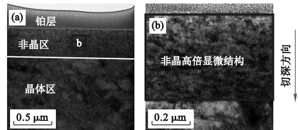
图 10 镍基单晶高温合金非晶转变形貌
