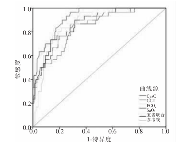
图 1 血清 CysC、GGT、PCO 2 、PO 2 、SaO 2 以及五者联合预测患者 COPD 重度病情的 ROC 曲线
