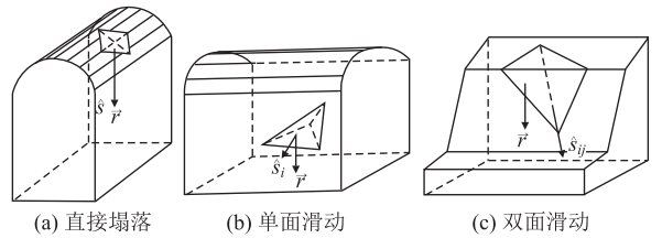
图 4 块体的运动模式
