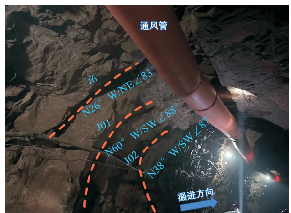
图 3 现场勘探平洞内几组优势结构面发育情况
