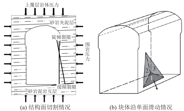
图 6 边墙单面剪切滑移-掉块模式
