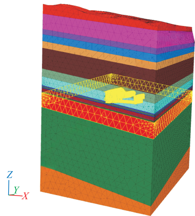
图 10 三维数值模型分层构建示意图
