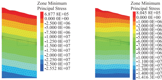
图 11 最大主应力分布和最小主应力分布图
