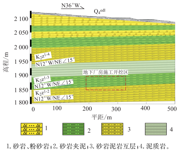
图 1 拟建地下厂房区工程地质剖面示意图
