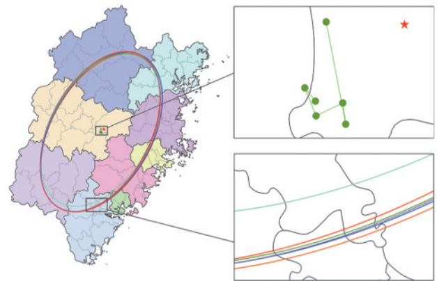
·森林生态系统服务价值重心 □县级行政区 □标准椭圆差2003年 *福建省几何重心 □市级行政区 □标准椭圆差2000年 □标准椭圆差2013年 □标准椭圆差2023年 □标准椭圆差2008年 □标准椭圆差2018年 图7 福建省森林生态系统服务价值标准差椭圆及重心移动轨迹 Fig. 7 Standard deviational ellipse and gravity center trajectory of forest ecosystem service value in Fujian Province
