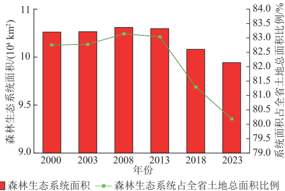
图 2 2000—2023 年福建省森林生态系统面积及占全省土地总面积比例
