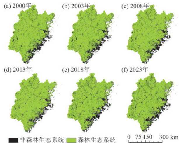
图 3 福建省不同时期森林生态系统分布
