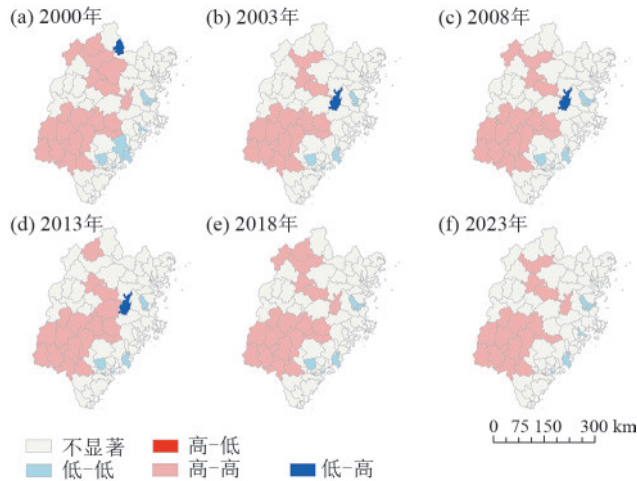
图 8 福建省森林生态系统服务价值 LISA 聚集图
