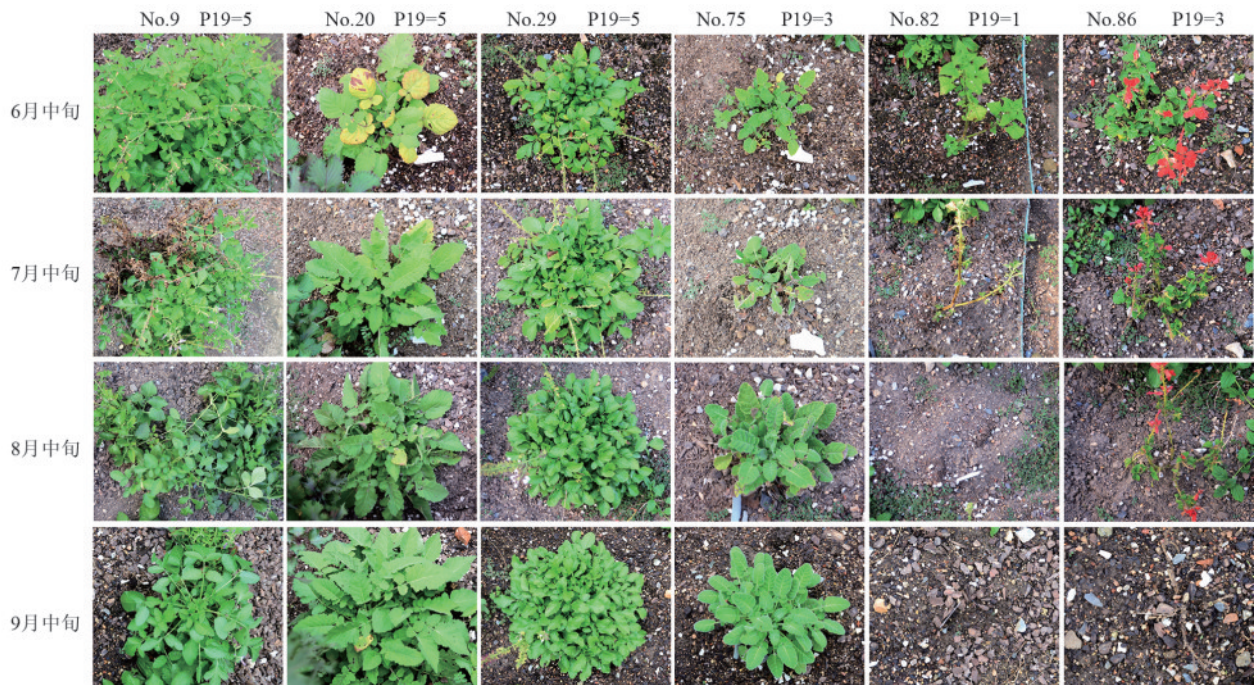
图1 示例6种(品种)鼠尾草在上海地区的越夏能力
