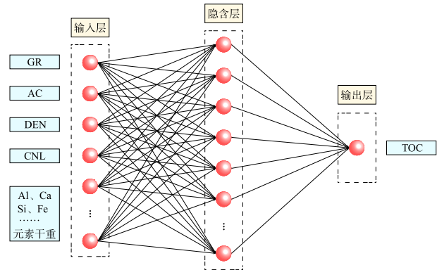
图 7 桂中坳陷鹿寨组一段 BP 神经网络预测 TOC 含量拓扑结构
