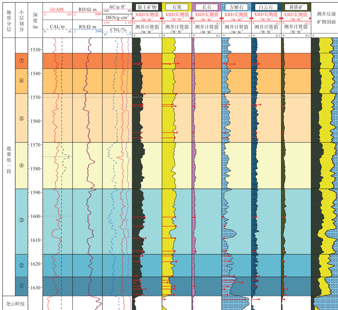
图 5 桂融页 1 井鹿寨组一段页岩矿物组分测井识别结果
