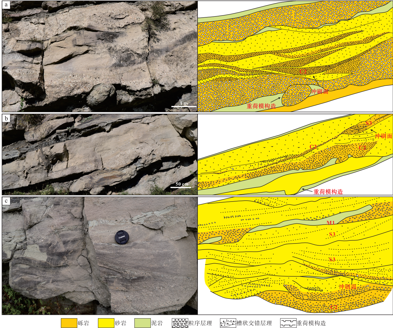
a—高密度浊流水道；b—高密度浊流水道；c—牵引流主控水下分流河道
