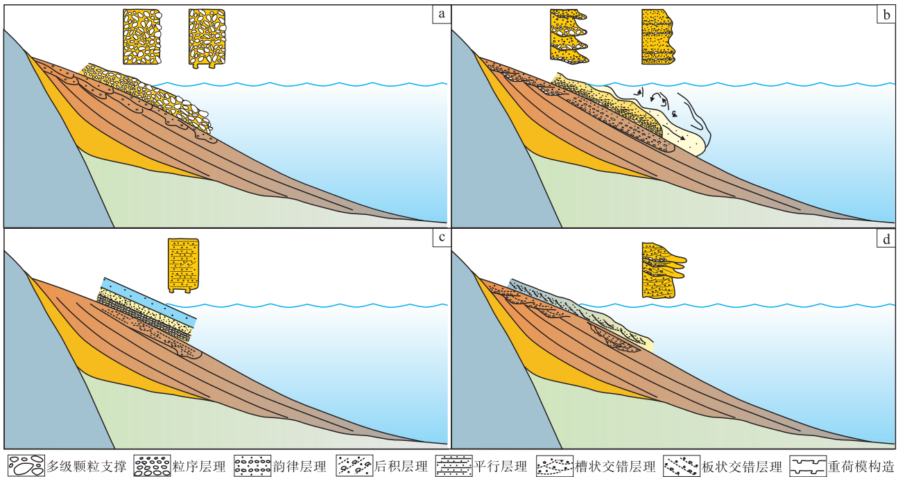
a—碎屑流建造期；b—洪流建造期；c—片流建造期；d—间洪期
