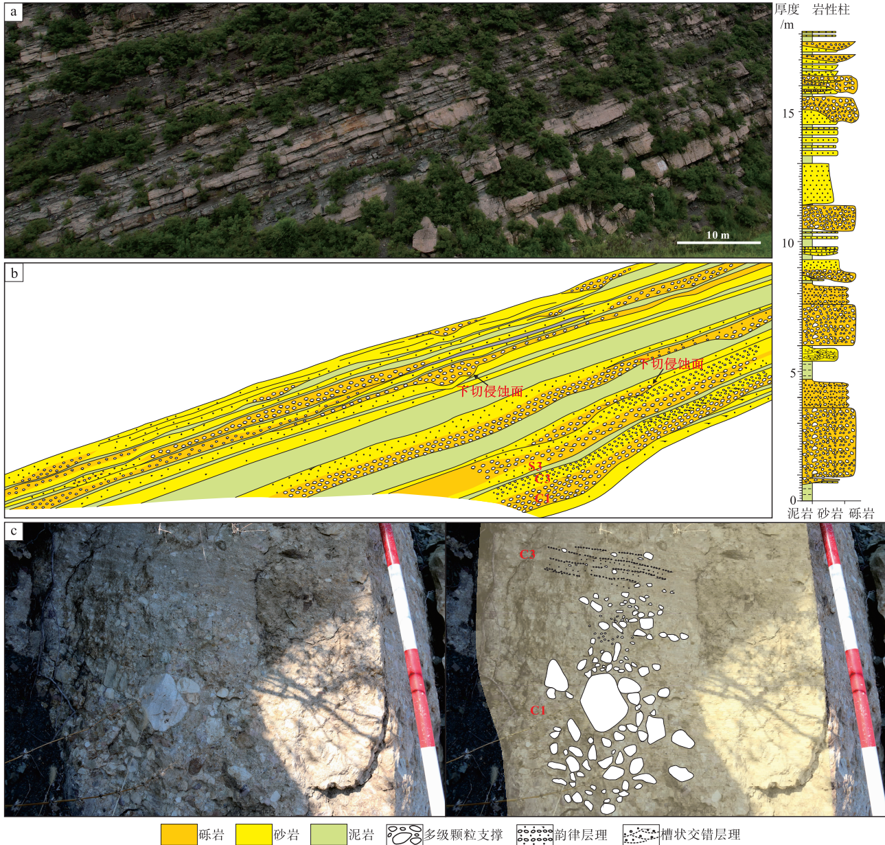
a—扇三角洲前缘典型露头照片；b—扇三角洲前缘砂砾岩体解释；c—朵体沉积特征 图 11 滦平盆地下白垩统西瓜园组桑园剖面扇三角洲前缘剖面解释 ( I )
