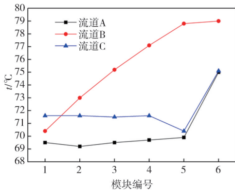
图4 3种冷板功率模块的底板平均温度分布曲线
