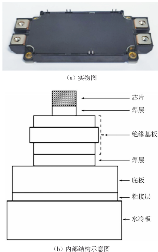
图 1 功率模块实物与内部结构示意图 Fig. 1 Power module and internal structure diagram
