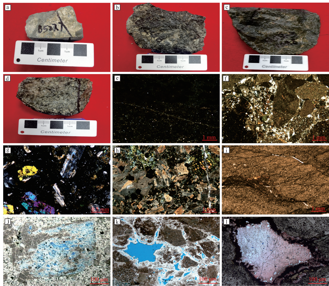
(a) 晶屑凝灰岩, 百527井, 1 133.22 m; (b) 凝灰质砂砾岩, 百527井, 1 183.00 m; (c) 透辉安山岩, 古53井, 1 164.80 m; (d) 蚀变闪长岩, 百107井, 1 130.00 m; (e) 晶屑凝灰岩岩石薄片, 百527井, 1 133.22 m; (f) 凝灰质砂砾岩岩石薄片, 百527井, 1 183.00 m; (g) 透辉安山岩岩石薄片, 古53井, 1 164.80 m; (h) 蚀变闪长岩岩石薄片, 百107井, 1 130.00 m; (i) 千枚状板岩岩石薄片, 古53井, 1 889.80 m; (j) 安山岩, 斑晶溶孔铸体薄片, 百107井, 1 130.32 m; (k) 凝灰质砂砾岩, 粒间溶孔铸体薄片, 百527井, 1 198.55 m; (l) 安山岩, 斑晶溶孔, 白杨1井, 3 470.00 m, 暗化边
