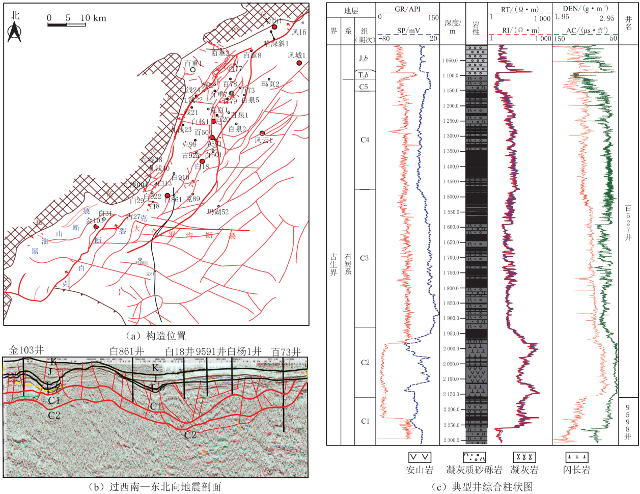
图 1 研究区构造位置、地震剖面 and 综合柱状图 Fig. 1 Tectonic location, seismic profile and comprehensive stratigraphic column of the study area
