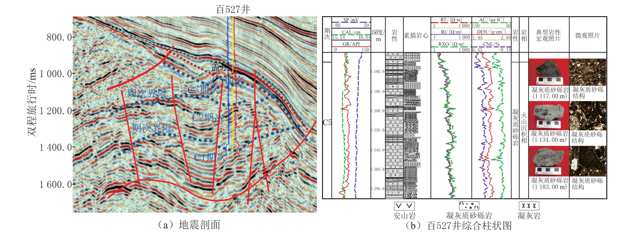
图 11 克百断裂带上盘石炭系 C5 期次 Fig. 11 Division of C5 sequences of the Carboniferous volcanic rocks on the hanging wall of the Kebai Fault Zone C1—C5 期次火山岩平面分布范围逐渐减小,与研究区呈两边高、中间低分布和 C2—C5 期次逐层超
