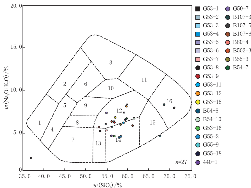
1. 霞岩; 2. 响岩质霞岩; 3. 响岩; 4. 碧玄岩; 5. 碱玄岩; 6. 响岩质碱玄岩; 7. 玄武岩和苦橄玄武岩; 8. 夏威夷岩; 9. 橄榄粗安岩; 10. 粗安岩 (歪长粗面岩); 11. 粗面岩; 12. 粗面安山岩; 13. 玄武安山岩; 14. 安山岩; 15. 英安岩; 16. 流纹岩 图 3 克百断裂带上盘石炭系火山岩全碱—硅图解(据文献[25]修改) Fig. 3 TAS diagram of the Carboniferous volcanic rocks on the hanging wall of the Kebai Fault Zone(modified by reference[25])
