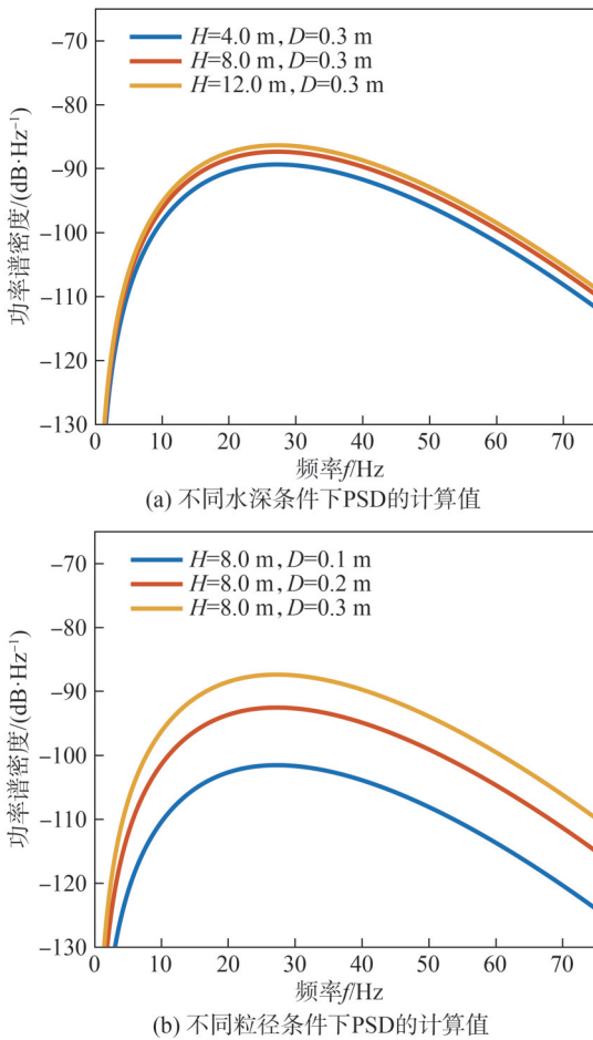
图5 不同水深与粒径条件下推移质功率谱密度 PSD 模型计算值
