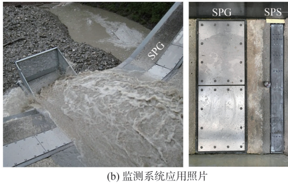
图 1 冲击板/管式推移质声震监测系统 [39] Fig. 1 Acoustic impact plate or pipe bedload monitoring systems [39] 1.1.2 冲击管/柱式监测系统
