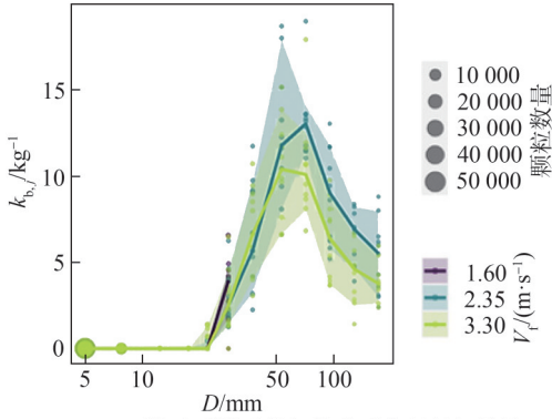
(b) 脉冲质量系数与推移质粒径的相关性
