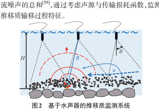
图 2 基于水听器的推移质监测系统 Fig. 2 Bedload monitoring system based on hydrophones 1.1.4 地震仪系统
