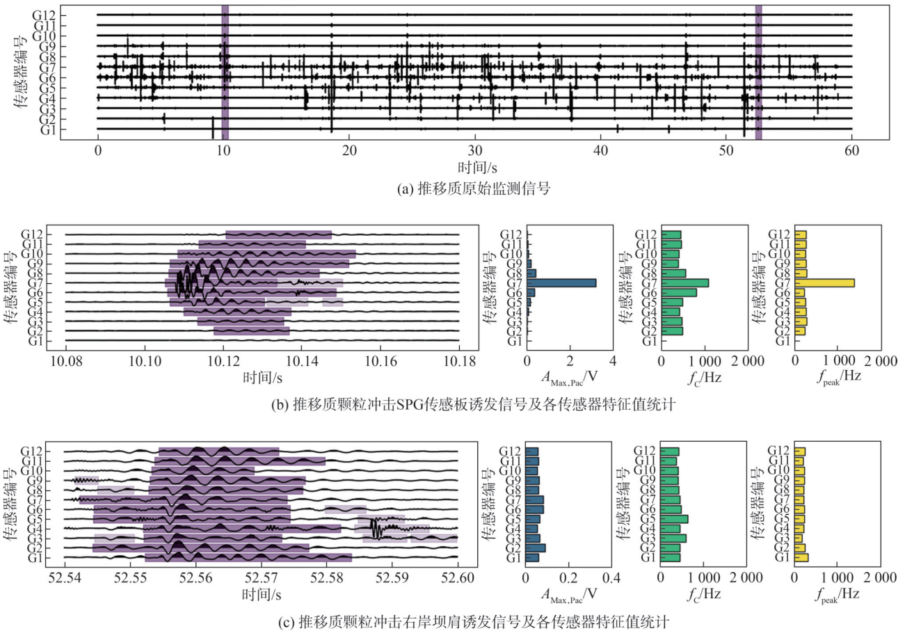
图6 瑞士Navisence山区河流推移质监测信号 [43]
