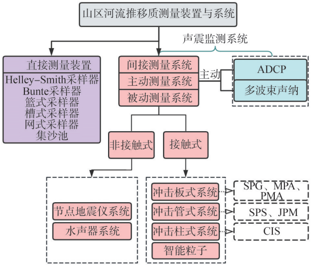
图 3 山区河流推移质输移采样装置与监测系统
