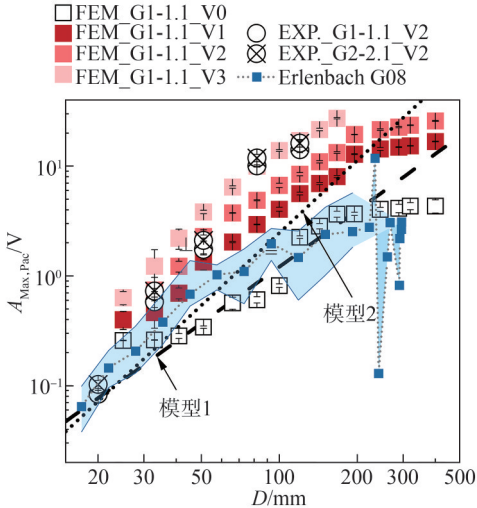
(a) 信号波包振幅与推移质粒径的相关性
