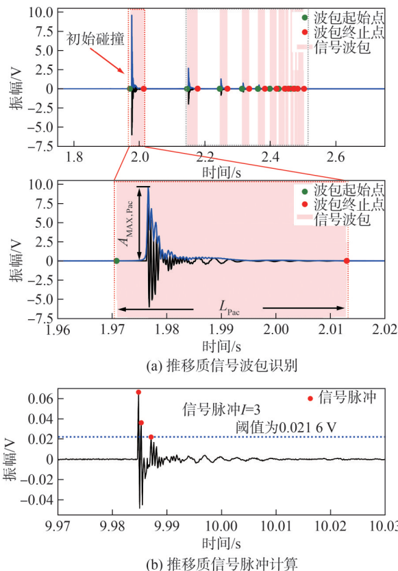
图4 推移质冲击SPG系统信号计算过程 [44]
