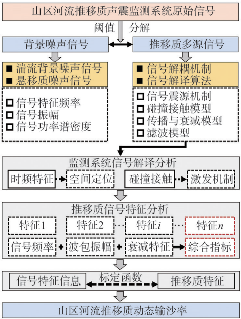
图 7 推移质输沙高频声震信号解译流程
